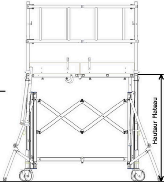
Plateauhöhe: 1550 mm
