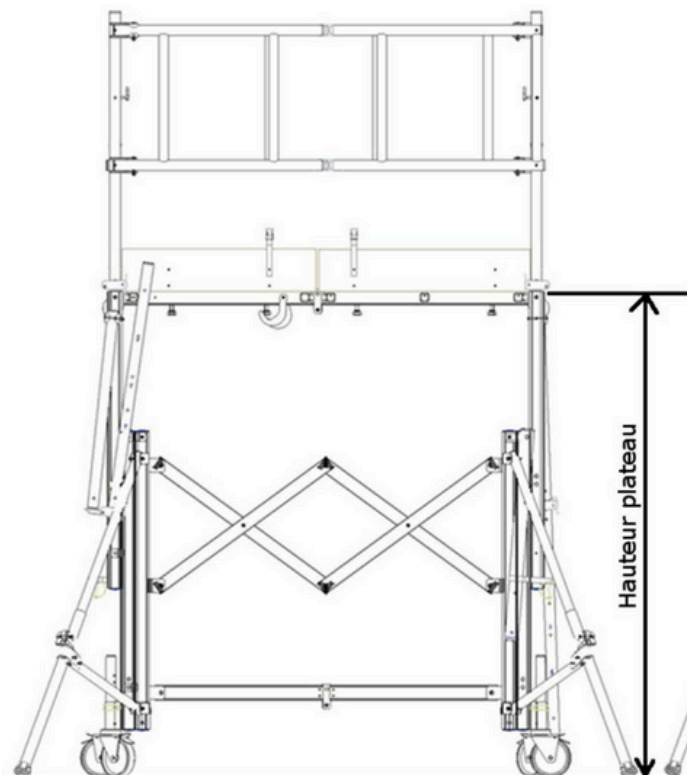
Plateauhöhe: 1800 mm
