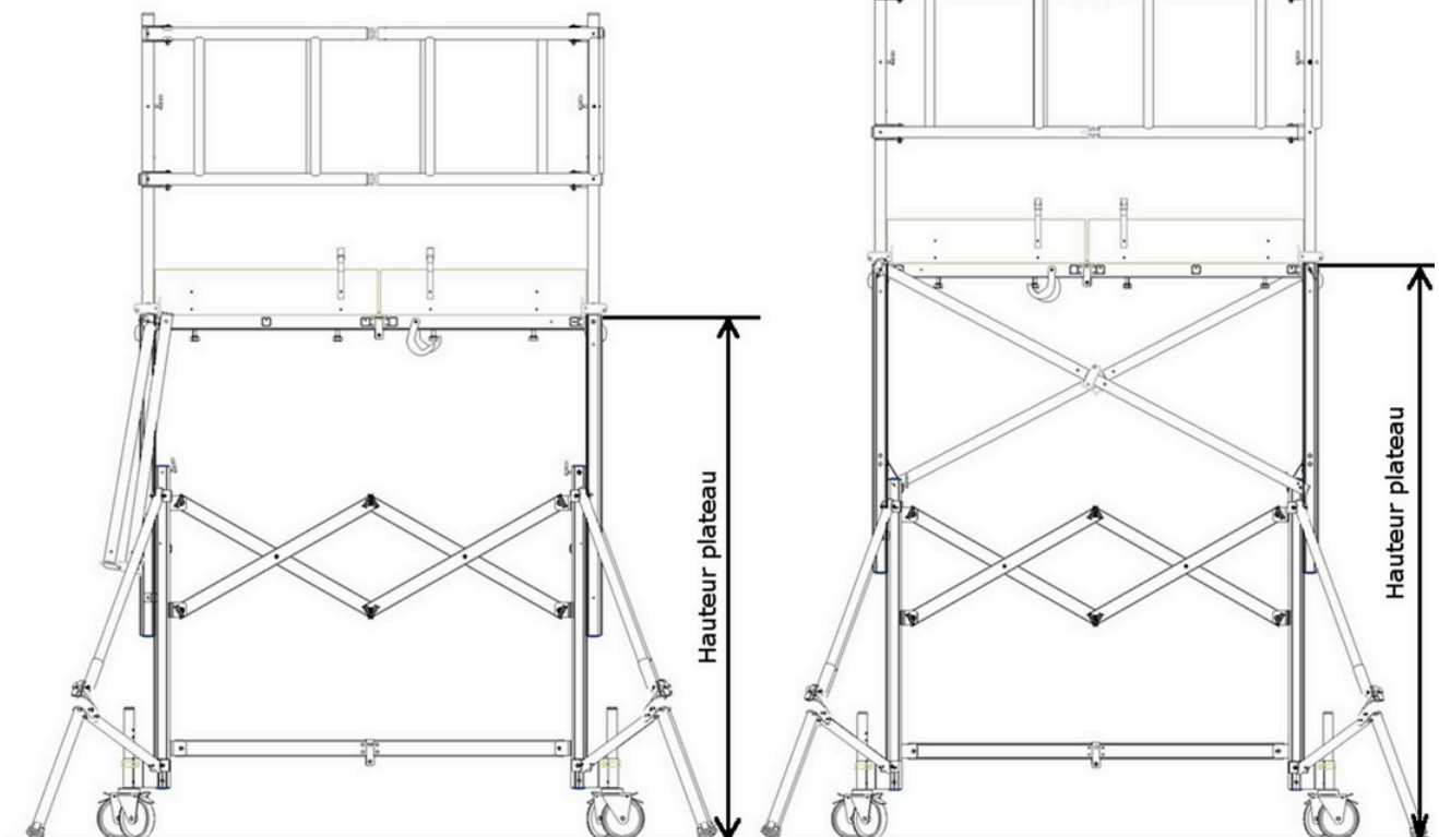
Plateauhöhe: 1800 mm
