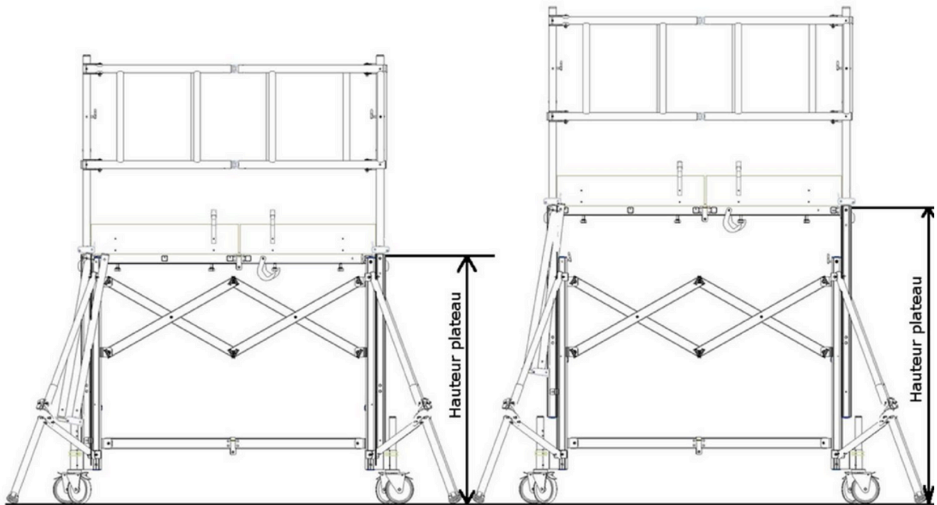
Plateauhöhe: 2050 mm
