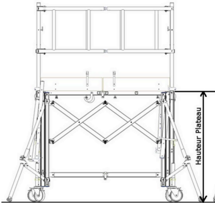
Plateauhöhe: 1300 mm
